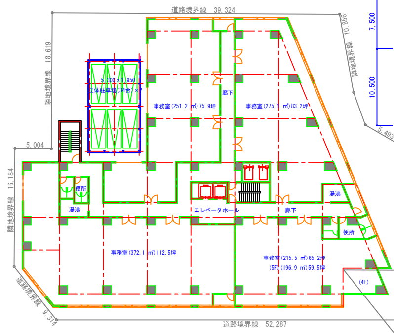
2~5階平面図 1/300
