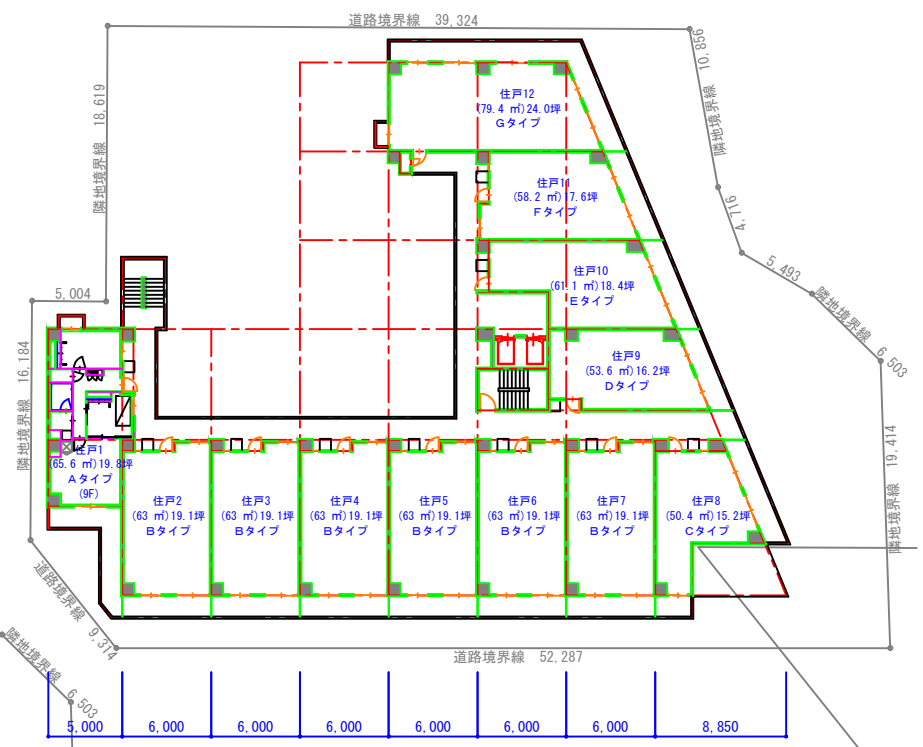
6~14階平面図 1/300
