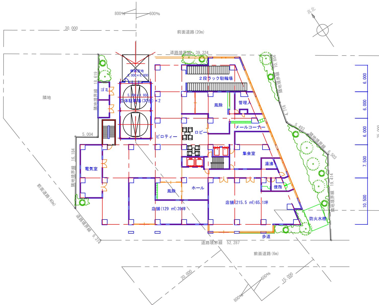
配置図・1階平面図 1/300
