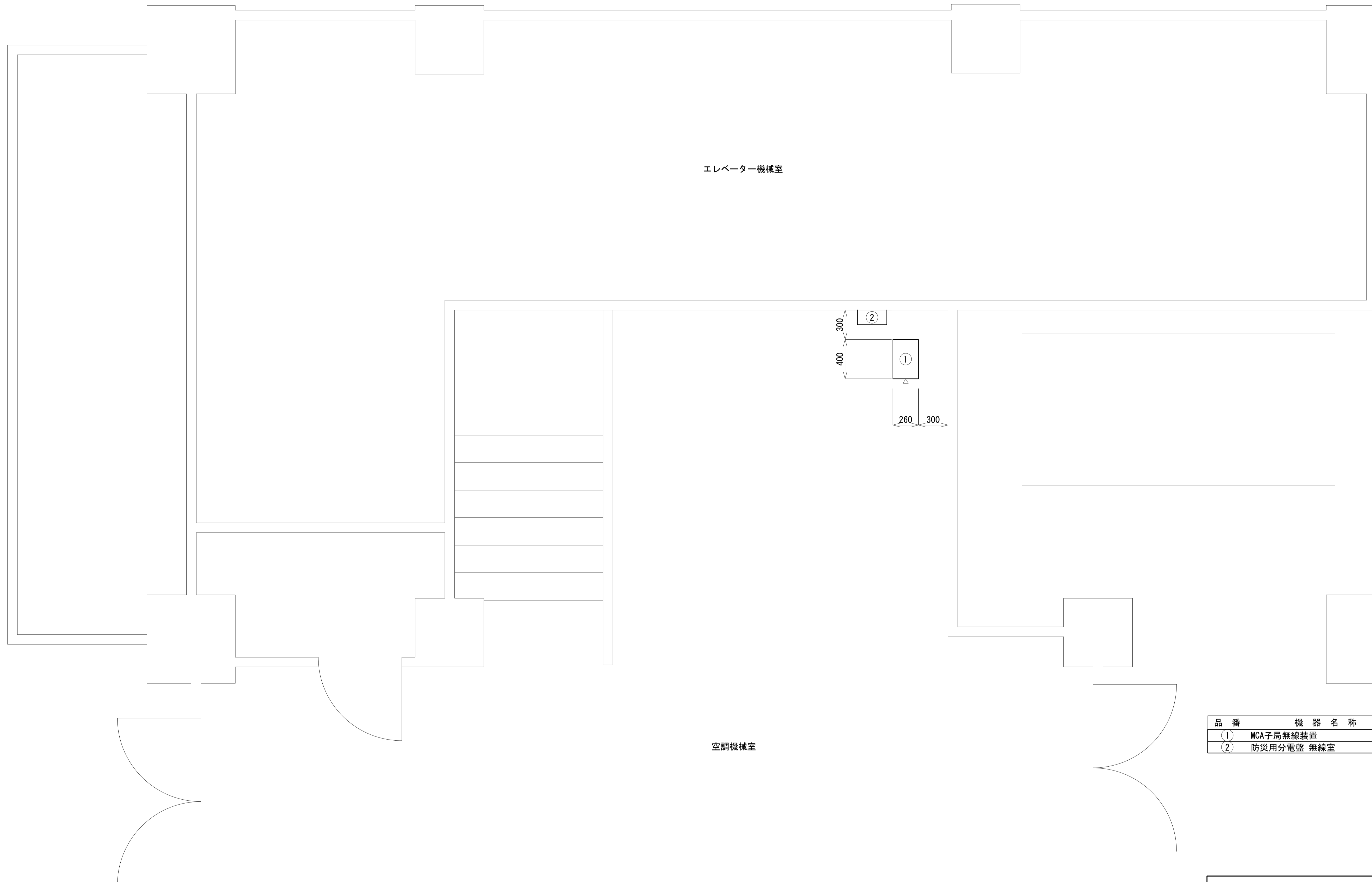
屋上1階 空調機械室 機器配置図(既設・撤去) S=1/20
