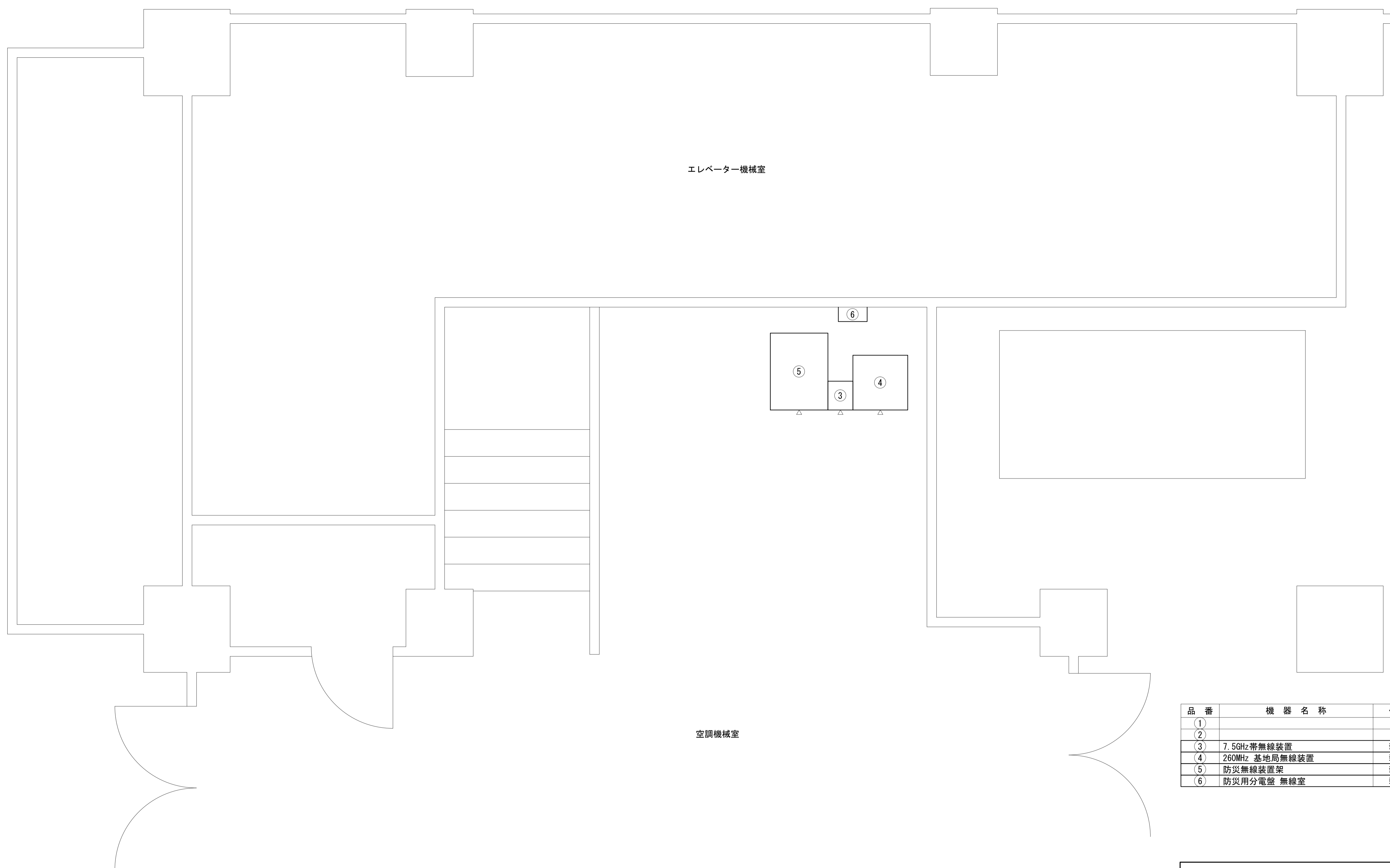
屋上1階 空調機械室 機器配置図(新設) S=1/20
