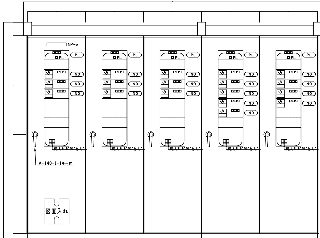
① 正面図
